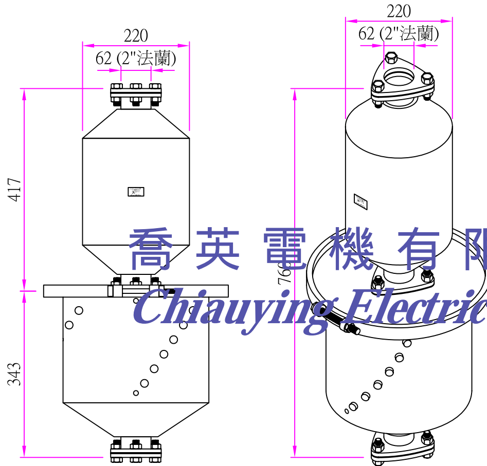
正視圖
